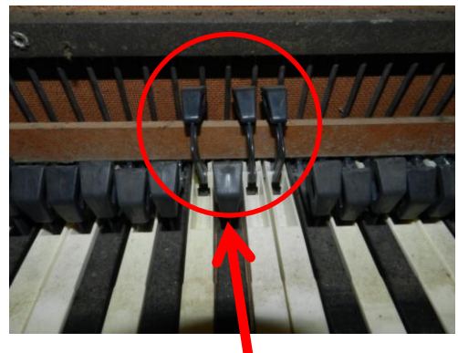
鍵盤が下がったままのところは ハンマーが上がったまま
